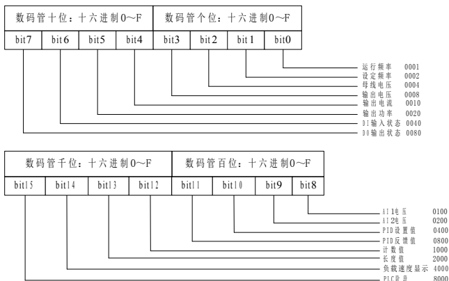
图 6-17. LED 运行显示位对应图
