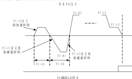
图6-28. 简易PLC示意图
