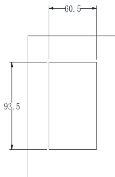
图2-8. 外引键盘带托盘安装开孔尺寸
