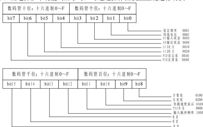
图 6-18. LED 停机显示对应图
