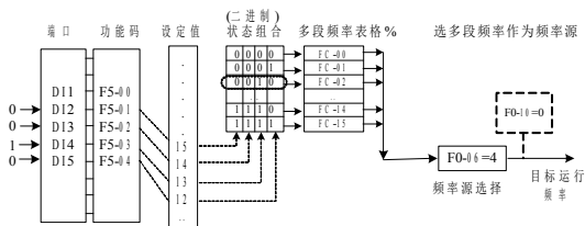
图4-21. 多段速控制示意图
