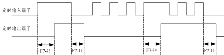
图 6-19. 定时器输入输出动作简图
