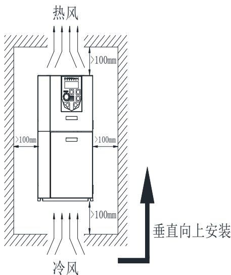
图3-1. 单体安装图
