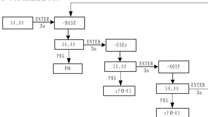
图 4-4. 菜单模式切换操作示意图
