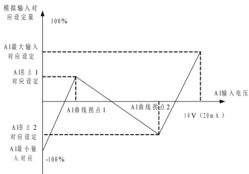
图6-29. 多点曲线对应示意图
