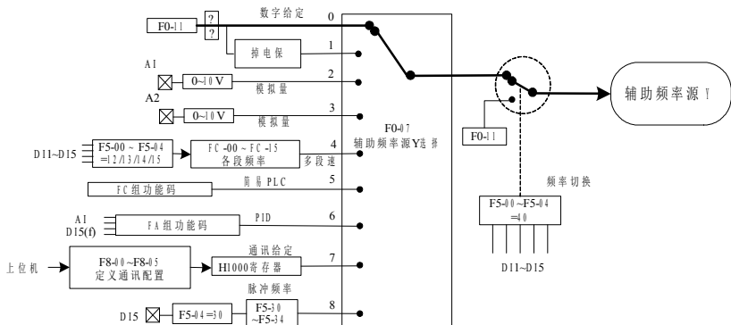
图4-18. 辅助频率源Y设置示意图
