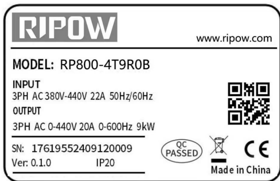
图2-2. 铭牌
