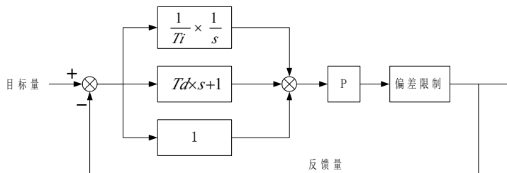
图6-23. 过程PID原理框图
