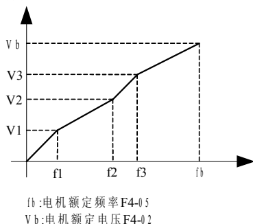
图 6-5. V/F 曲线设定示意图
