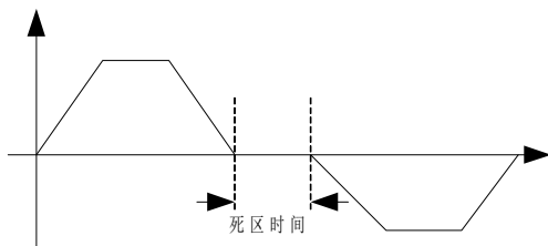
图 6-14. 正反转死区时间示意图
