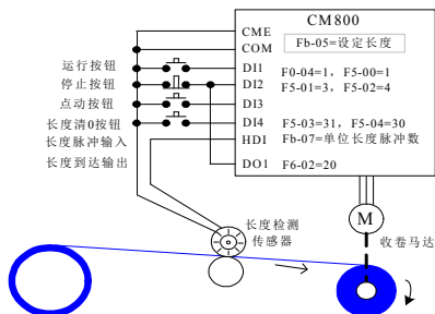
图 4-24. 定长控制功能常见应用举例
