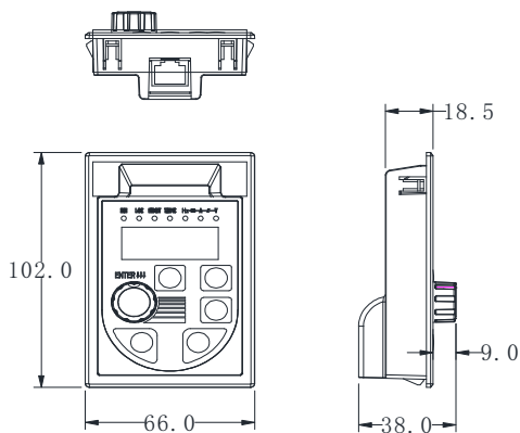
图2-7. 外引键盘带托盘安装尺寸图
