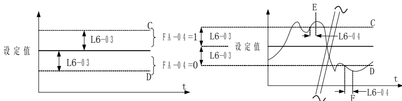
图6-32. 唤醒示意图
