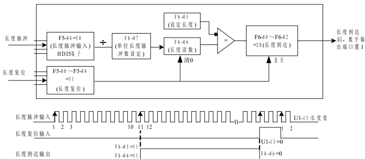
图 4-23. 定长控制模式功能码设置
