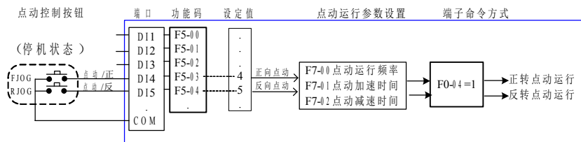
图4-16. DI方式点动参数设定示意图
