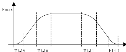
图 6-3. S 曲线加减速示意图
