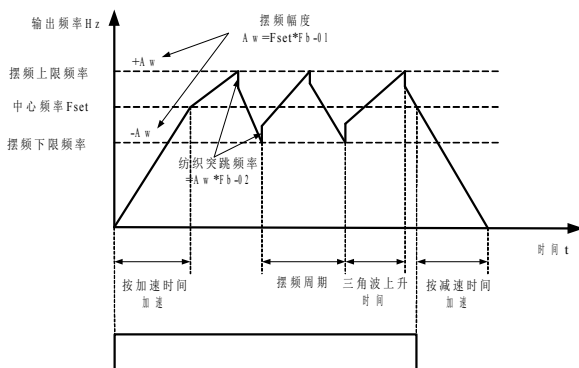
图6-26. 摆频工作示意图
