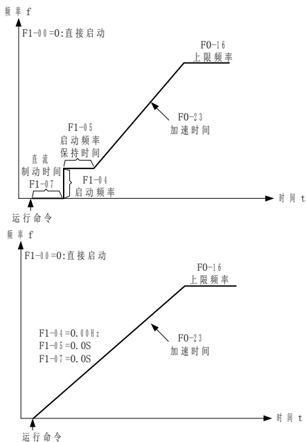
图4-11. 直接启动示意图
