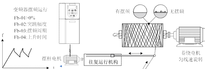
图4-20. 摆平运用设置示意图
