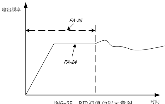
图6-25. PID初值功能示意图
