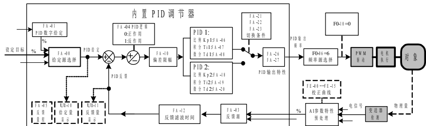
图4-19. 频率闭环控制示意图
