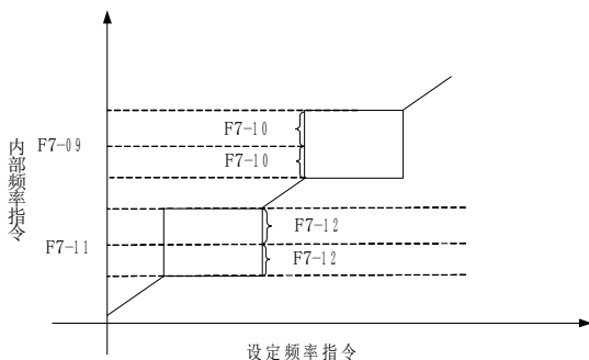
图 6-13. 跳跃频率示意图
