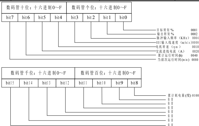
图 6-20. LED 运行显示位对应图
