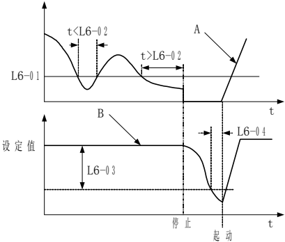
图6-31. 休眠过程频率图
