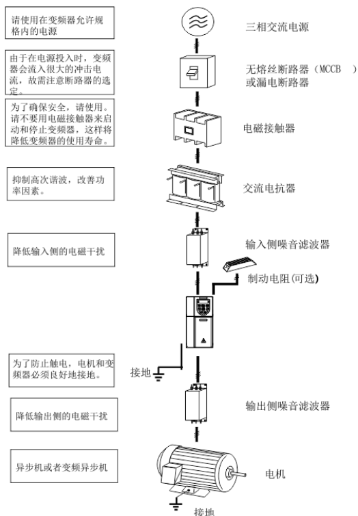
图 1. 与外围机器的连接示例
