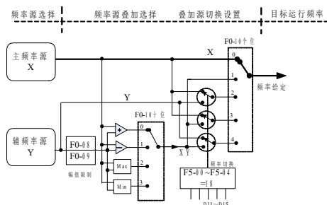
图6-1. 频率源叠加示意图
