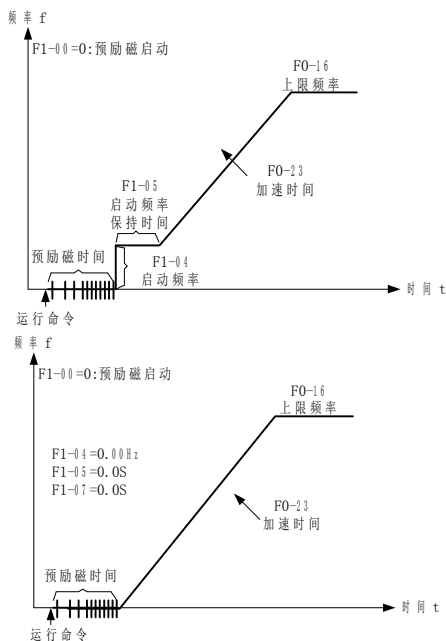
图4-12. 预励磁启动示意图
