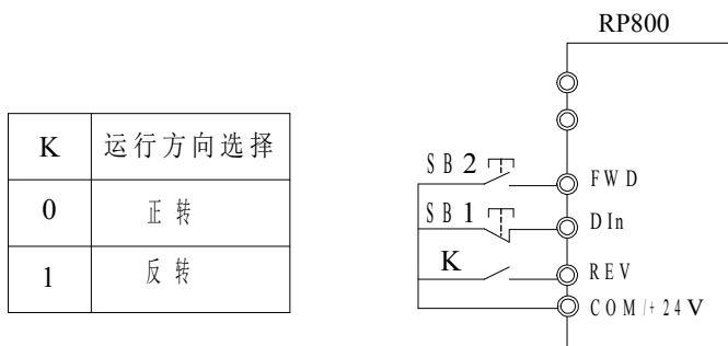
图 6-10. 三线式运转模式 2
