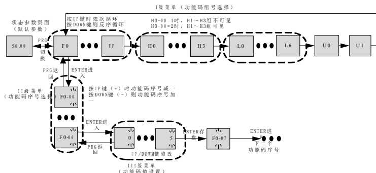
图4-2. 三级菜单操作流程
