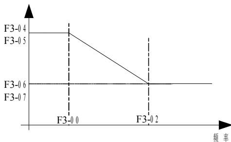
图 6-6. 速度环 PI 参数切换示意图
