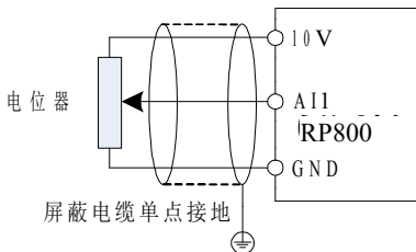
图 3-3. 模拟量输入端子接线示意图
