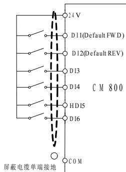
D1接线模式三：当DI拨码开关为PNP模式没有使用外部电源
