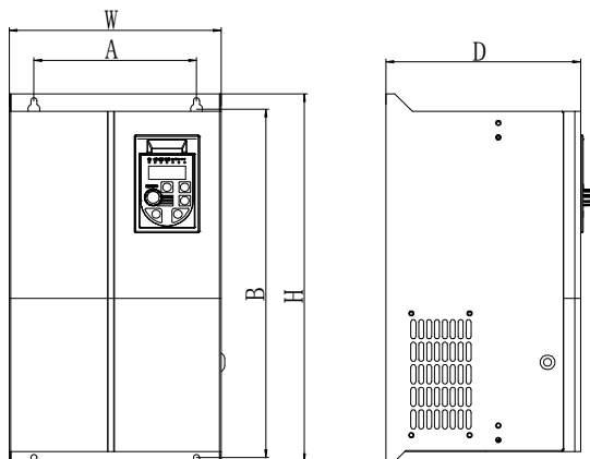
图 2-4. 30~75kW 钣金机箱尺寸及安装尺寸示意图
