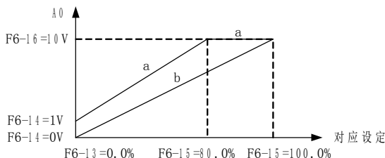
图6-12. 模拟输出上下限对应关系
