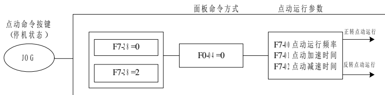
图4-15. 点动参数设定示意图
