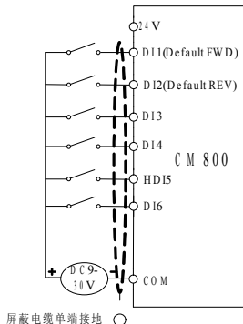
图3-4. 四种不同模式下数字输入端子接线图
