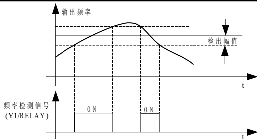
图 6-16. 频率到达检出幅值示意图
