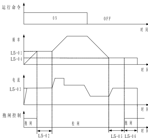
图6-30. 抱闸控制过程图
