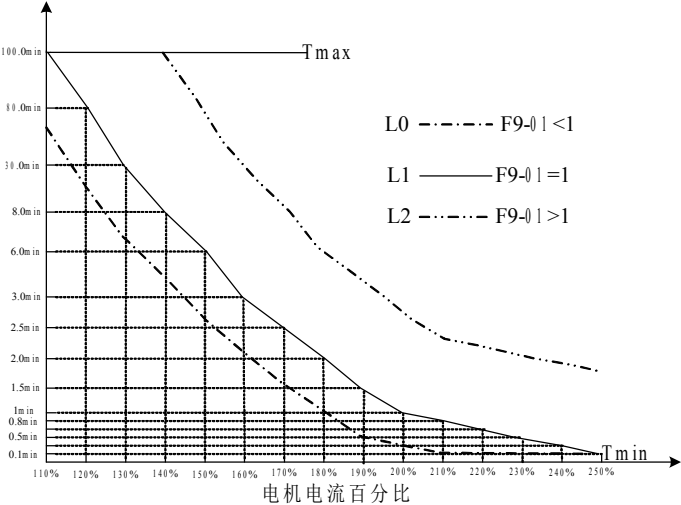
图6-21. 电机过载保护曲线
