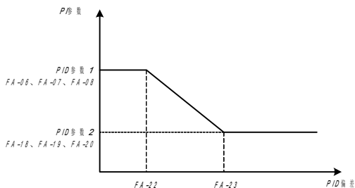
图6-24. PID参数切换
