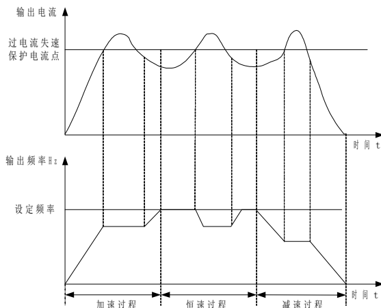
图6-22. 过流失速保护示意图
