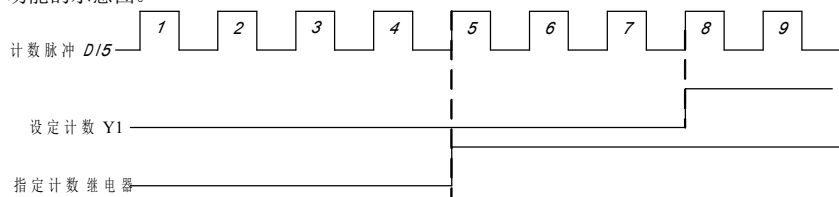
图6-27. 设定计数值给定和指定计数值给定示意图
