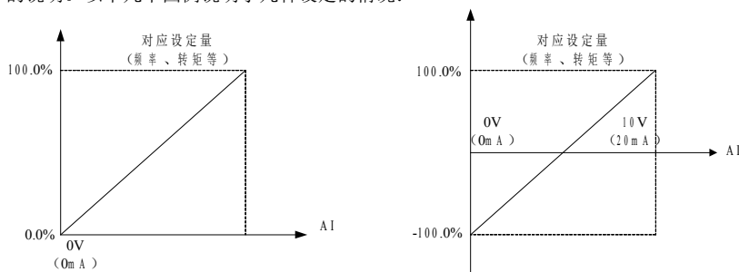
图 6-11. 模拟给定与设定量的对应关系
