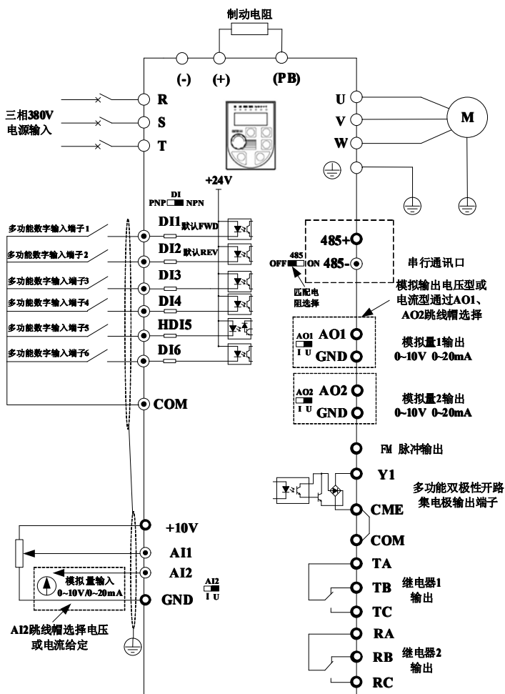
图3-2. 三相变频器（380V）11kW及以上（通用型）
