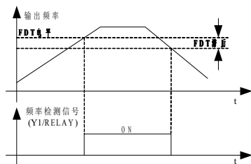
图 6-15. FDT 电平示意图
