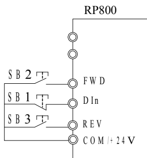
图 6-9. 三线式运转模式 1
