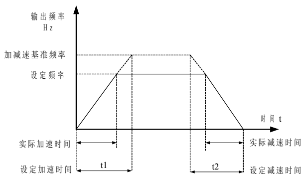
图6-2. 加减速时间示意图
