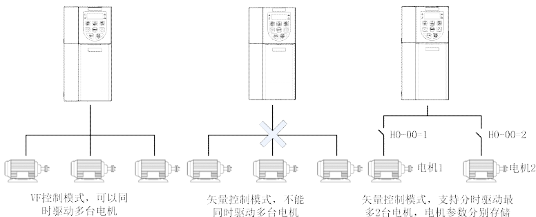
图 4-26. 多组电机的切换
